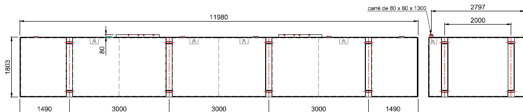
VUE SUR PONT
