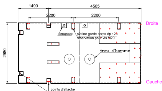
VUE SUR PONT
