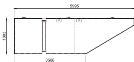
VUE SUR PONT
