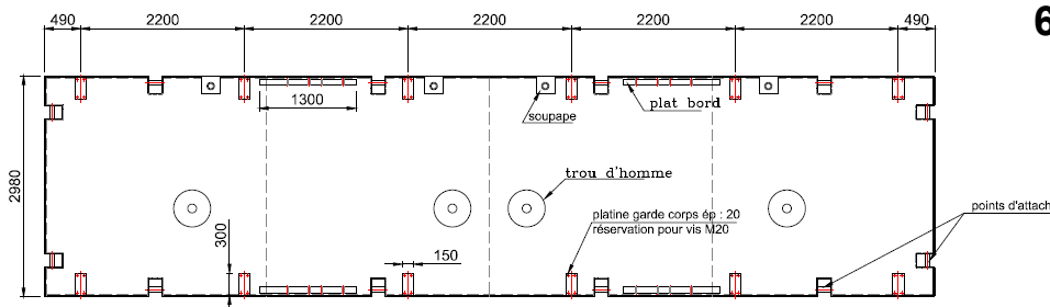
VUE SUR PONT
